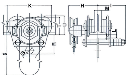
Mechanische loopkat GT-5
